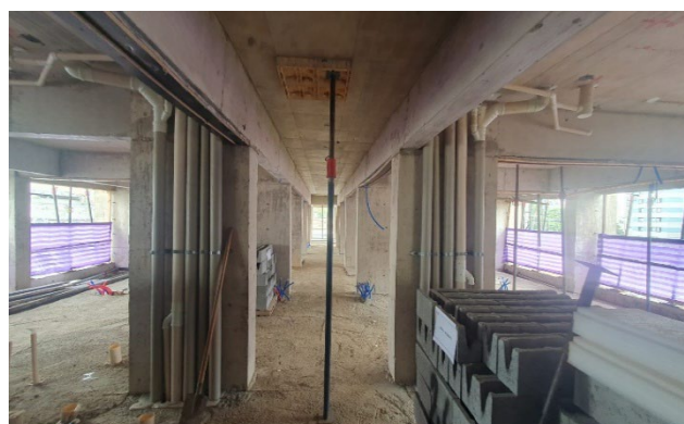
Estrutura e instalações – 2º Pavimento.
