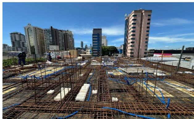
Armação vigas e laje 4º pavimento – Lado A..
