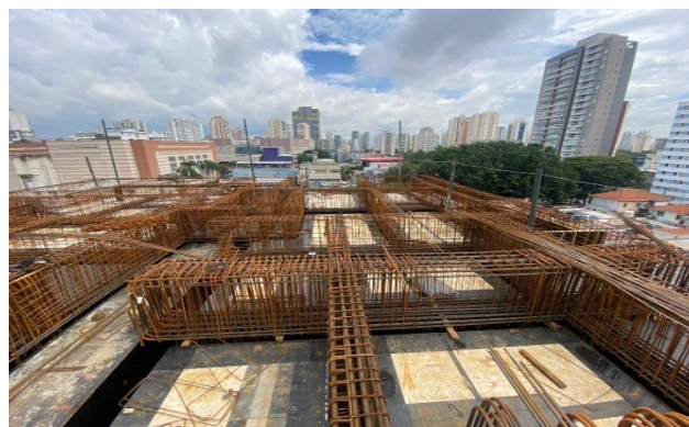
Armação vigas e laje 4º pavimento – Lado B.
