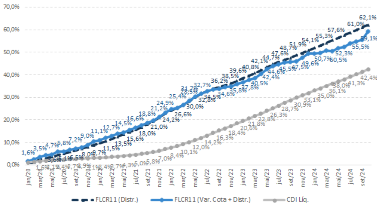
GRÁFICO 3: RENTABILIDADE ACUMULADA
