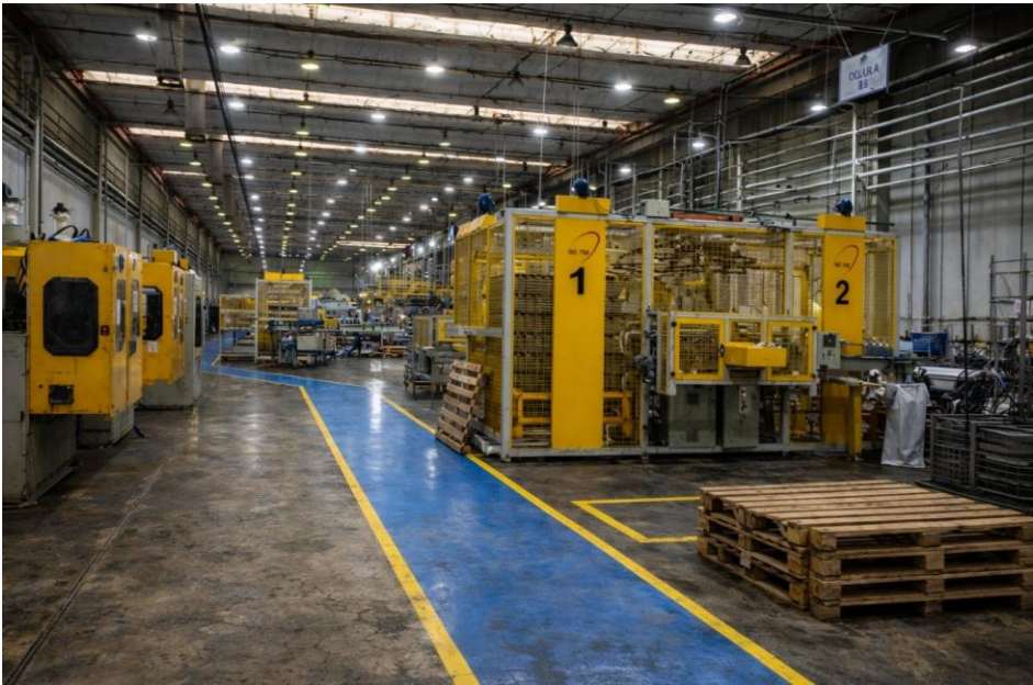
Vista interna do galpão industrial, com ocupação integral pela empresa Globalpack.
