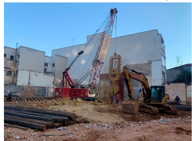
Execução de parede diafragma em agosto/24.
