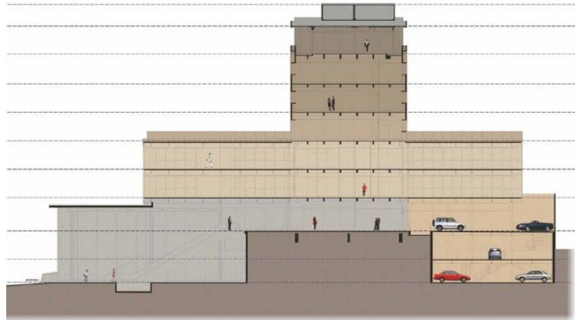
CORTE ESQUEMÁTICO DO EDIFÍCIO
