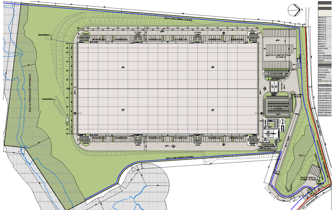
PLANTA DE IMPLANTAÇÃO GERAL DO PROJETO
