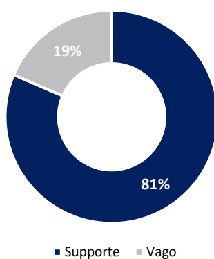
Gráfico 7: Ocupação Financeira
