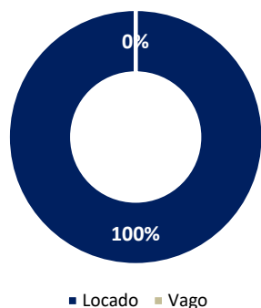
Gráfico 5: Ocupação Física
