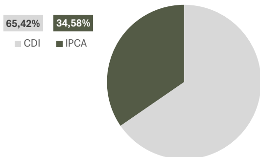
Gráfico 7 – Indexadores
