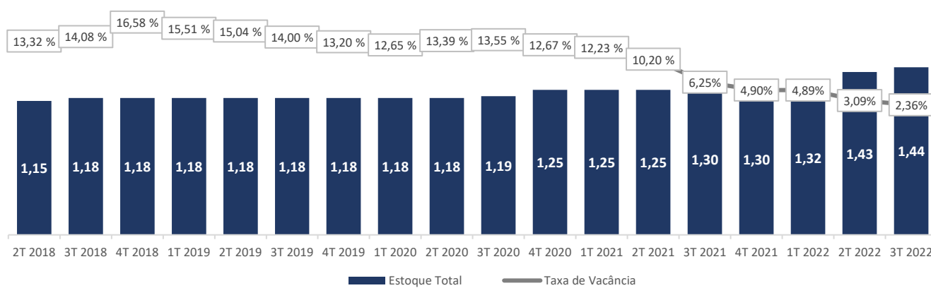
Gráfico 12: Inventário Existente (Milhão de m²) e Taxa de Vacância no Mercado Local 17
