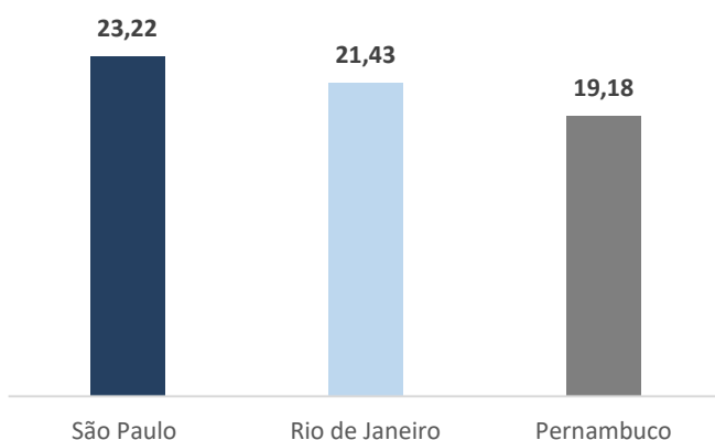
Gráfico 17: Preço Médio Pedido (R$/m 2 /mês) 17
