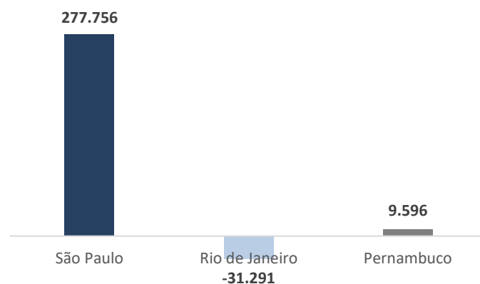
Gráfico 16: Absorção Líquida (m 2 ) 17
