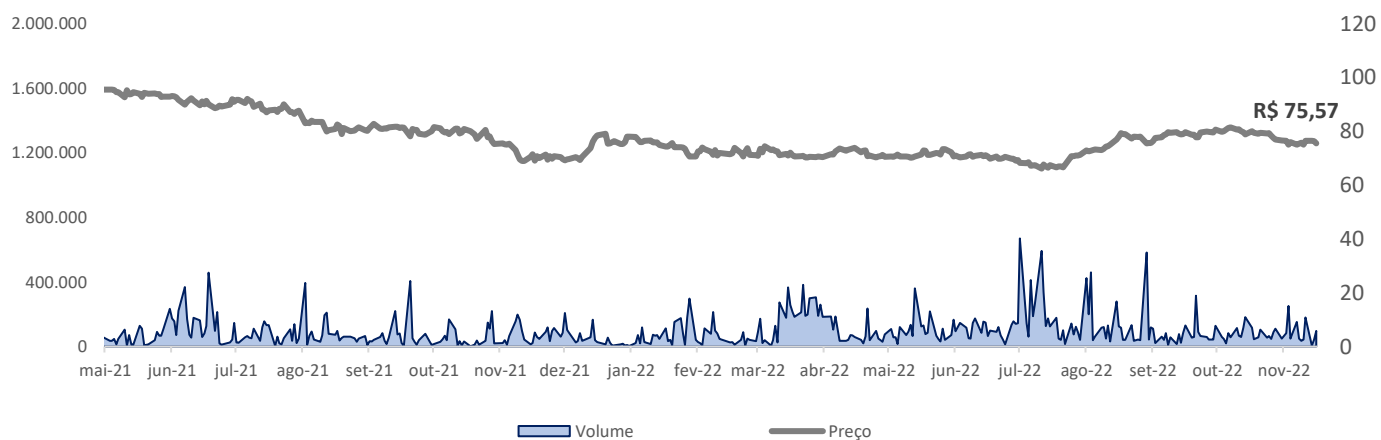
Gráfico 2: Preço e Volume Negociado desde o IPO do Fundo (valores em R$)
