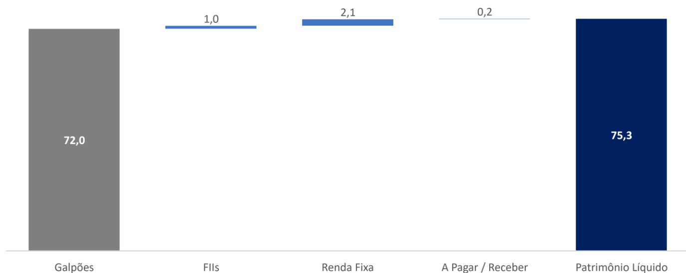
Gráfico 4: Bridge Patrimônio Líquido (valores em R$ mm)
