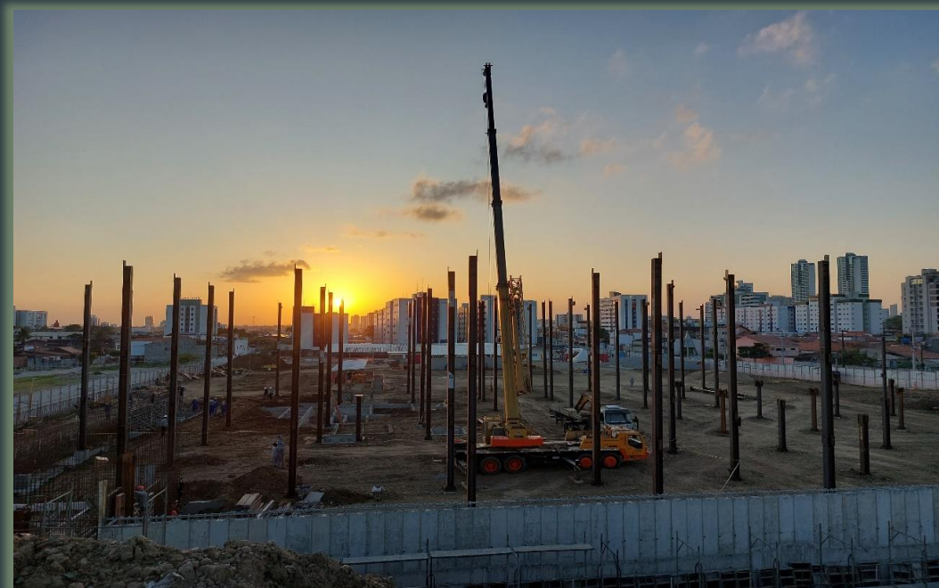
Montagem dos pilares das estruturas metálicas.
