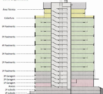
Corte Esquemático
