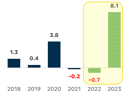
PIB Agropecuário
